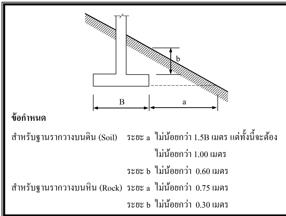
รูปที่ 2 ข้อกำหนดสำหรับการก่อสร้างฐานรากบนพื้นที่ลาดเอียง
