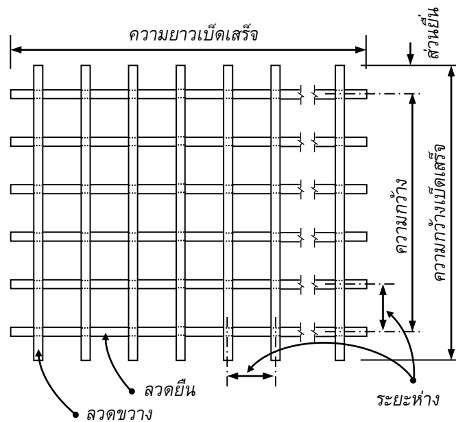
รูปที่ 1 ส่วนต่างๆ ของตะแกรงหลักกล้าลวดเดี่ยว
