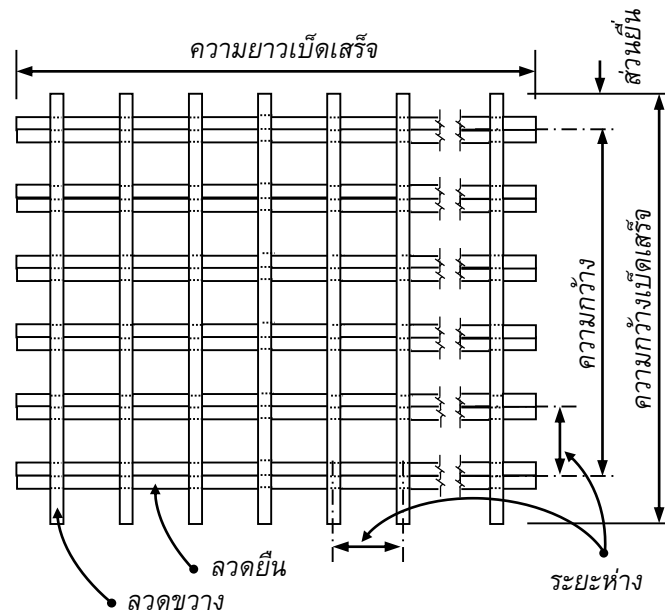
รูปที่ 2 ส่วนต่างๆ ของตะแกรงเหล็กกล้าลวดคู่ (ข้อ 4.5)
