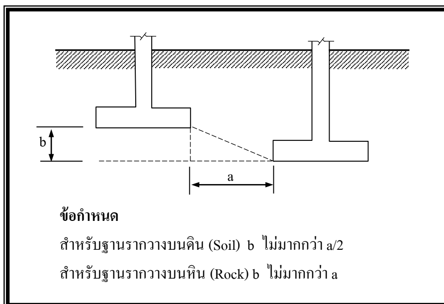
รูปที่ 1 ข้อกำหนดสำหรับการก่อสร้างฐานรากที่มีความลึกต่างกัน (ข้อ 4.1.3)
