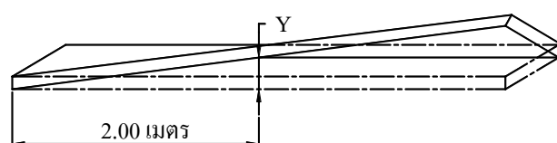
รูปที่ 7 การเสีรูปสูงสุดที่ยอมให้ในช่วงความยาว 2 เมตร
