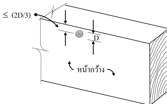
รูปที่ 1 เกณฑ์การจำแนกตาไม้ที่ขอบของหน้ากว้างขององค์อาคารรับแรงดัด
