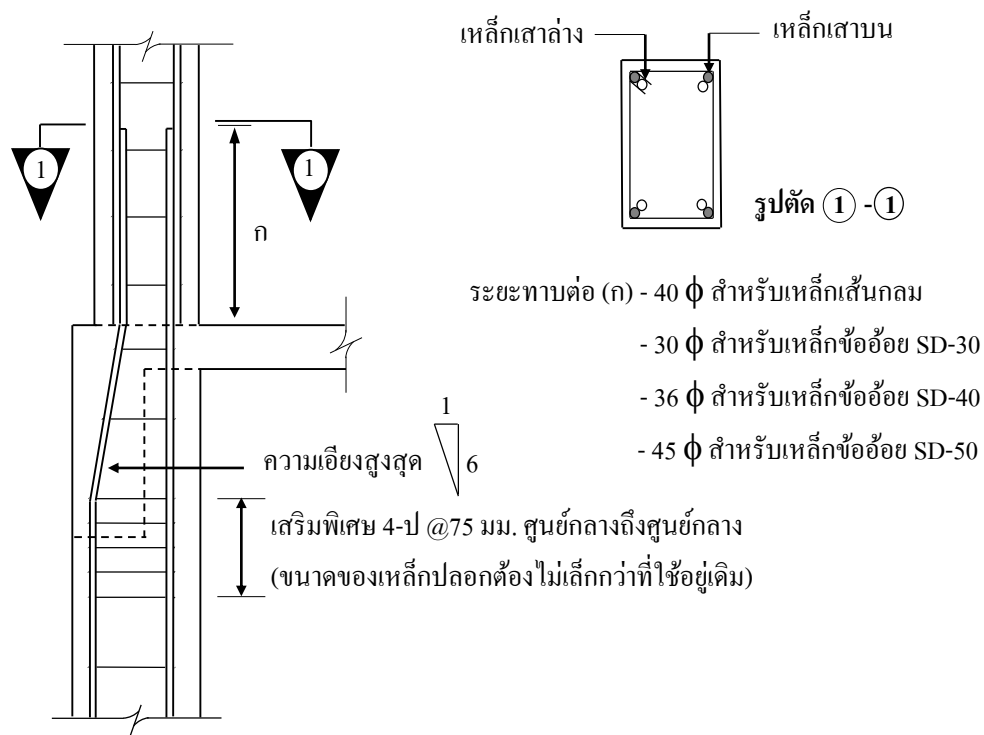
รูปที่ 6 กรณีเสามีหน้าตัดไม่เท่ากันศูนย์เยื้องกัน
